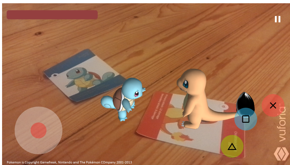
Obrázek C.2: Hra
