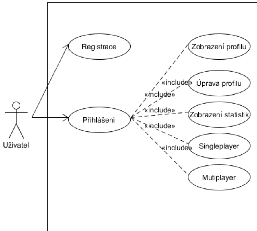
Obrázek 2.1: Diagram případů užití
