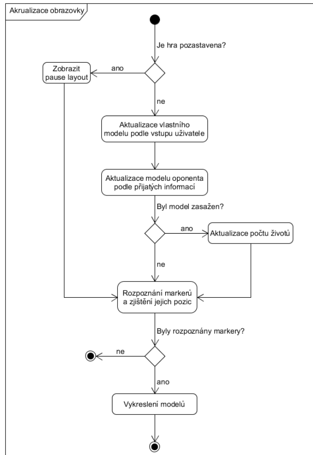
Obrázek 3.1: Diagram: Vykreslování rozšířené reality
