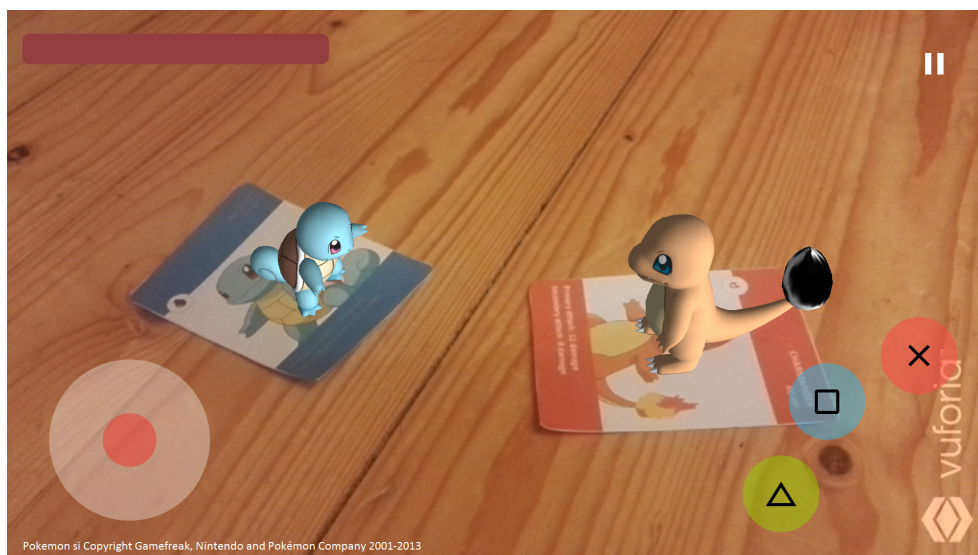
Obrázek C.1: Hra
